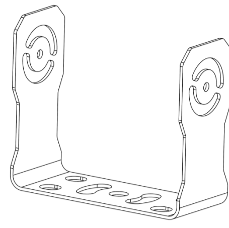
Bevestigingsbeugel x 1
